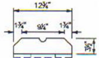
TOP BRACE
